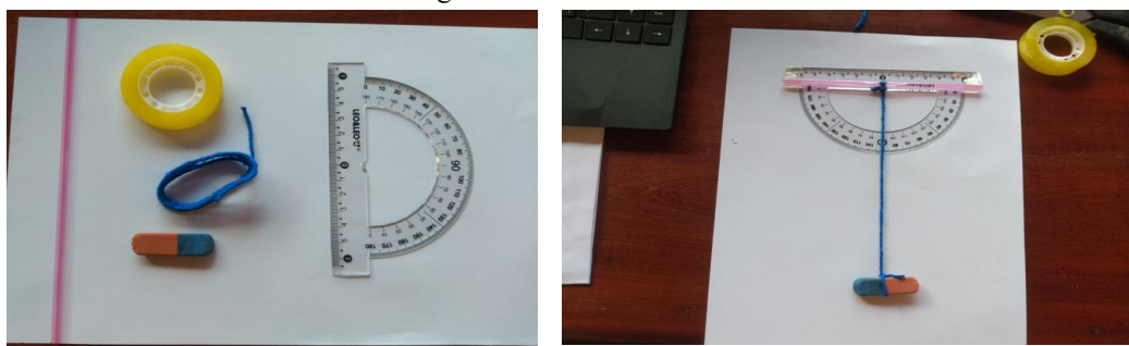
Figura 9 – teodolito caseiro
